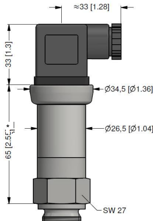
G1/2" DIN 3852 / ISO 4400
