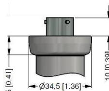
Binder Seria 723 7-pin (IP 67)
